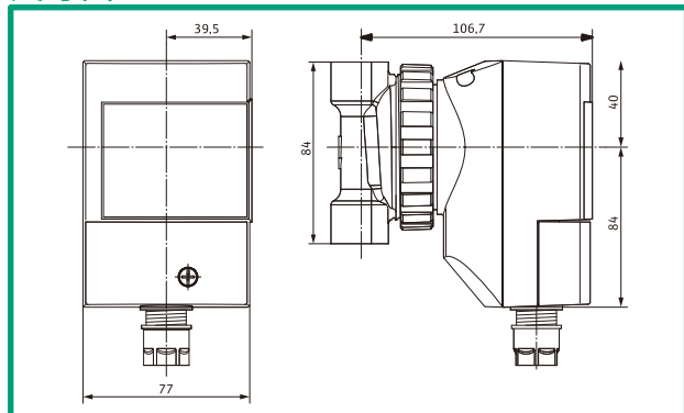
尺寸圖 C
