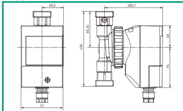
尺寸圖 D
