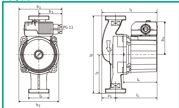
尺寸圖 F
