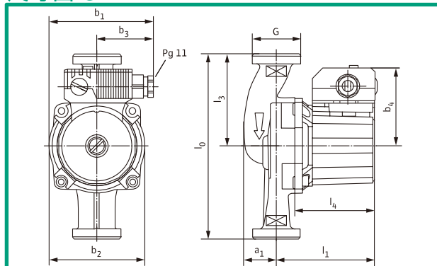
尺寸圖 G
