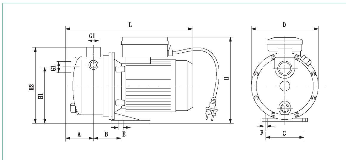
Jet WJ..X尺寸圖
