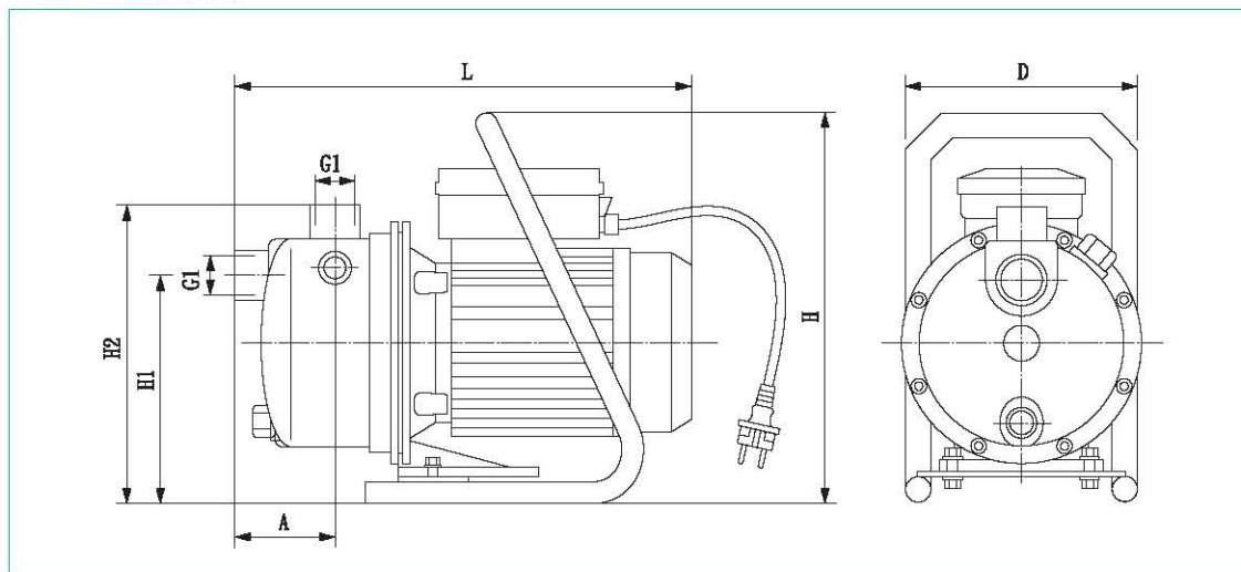
Jet WJ尺寸圖
